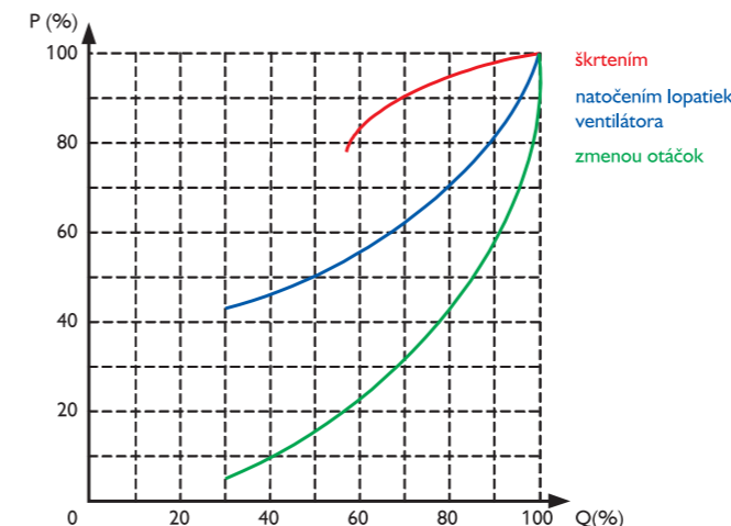
Príkon motora pri rôznych spôsoboch regulácie ventilátora
