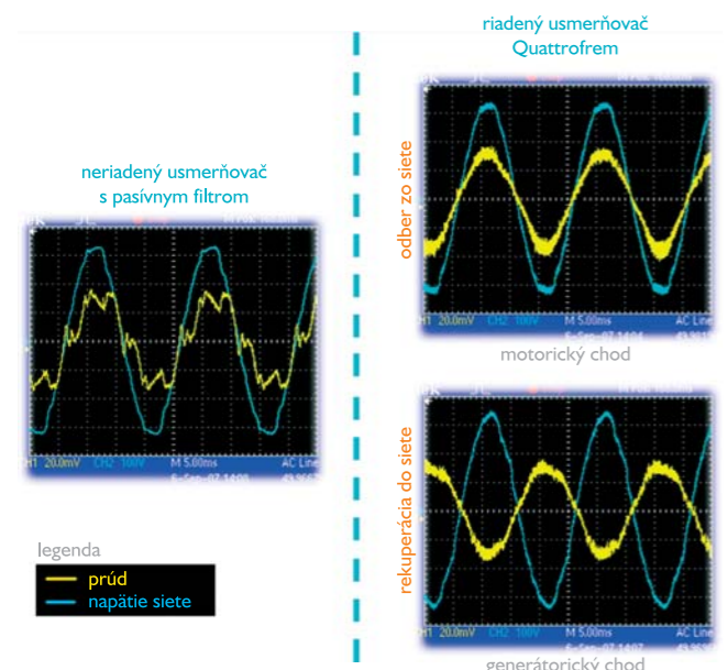
Obr.1 Priebehy vstupných prúdov (merané s motorom s výkonom 18,5 kW pri plnom zaťažení)
