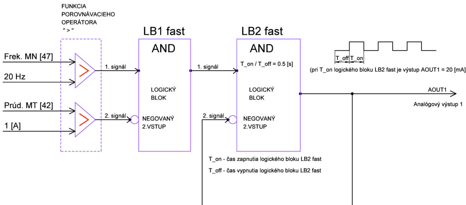
Bloková schéma vyhodnocovania vstupných podmienok pomocou logických blokov
