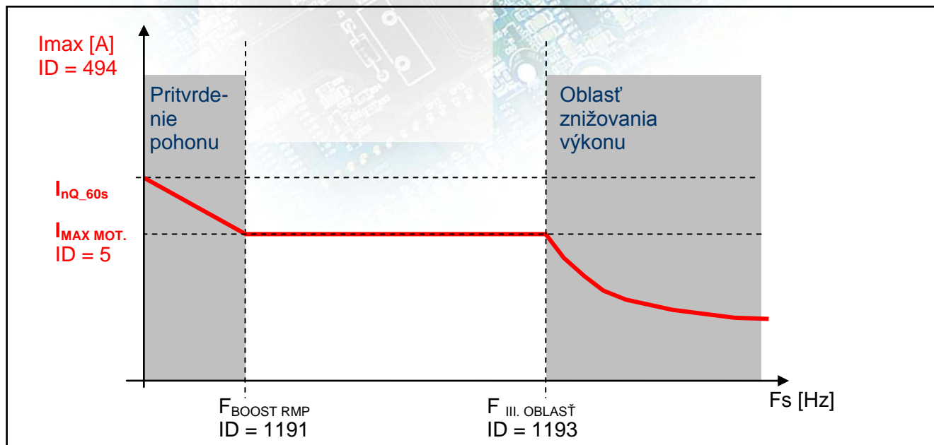
Obrázok: Špecifické prípady úpravy hranice maximálneho prúdu:
