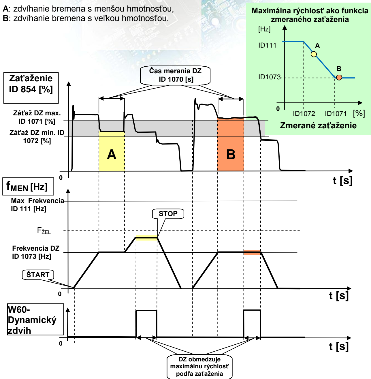
Obrázok dole: Princíp činnosti funkcie „Dynamický zdvih“.
