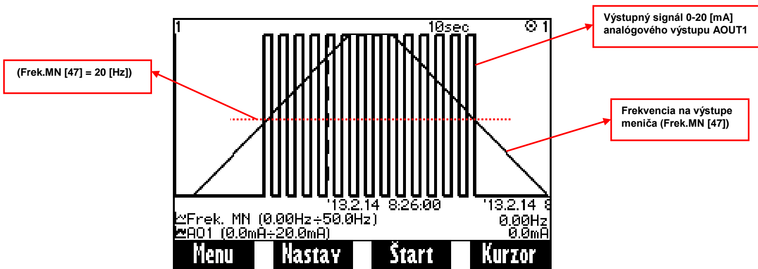
Priebeh veličín
